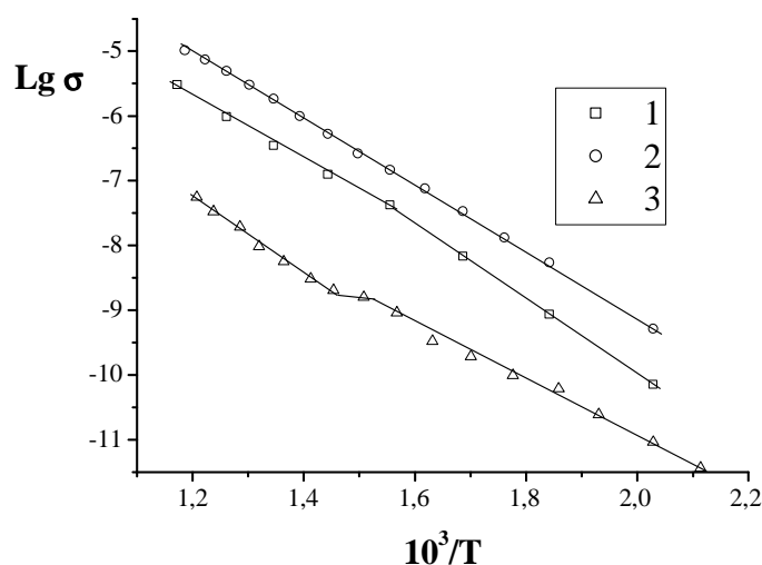
Рис. 2. Залежність \text{Lg}(\sigma) - 1000/t \text{ (K)} : 1 – \text{LiInP}_2\text{O}_7 ; 2 – \text{LiIn}_{0,95}\text{Mn}_{0,05}\text{P}_2\text{O}_7 ; 3 – \text{NaIn}_{0,98}\text{Mn}_{0,02}\text{P}_2\text{O}_7
