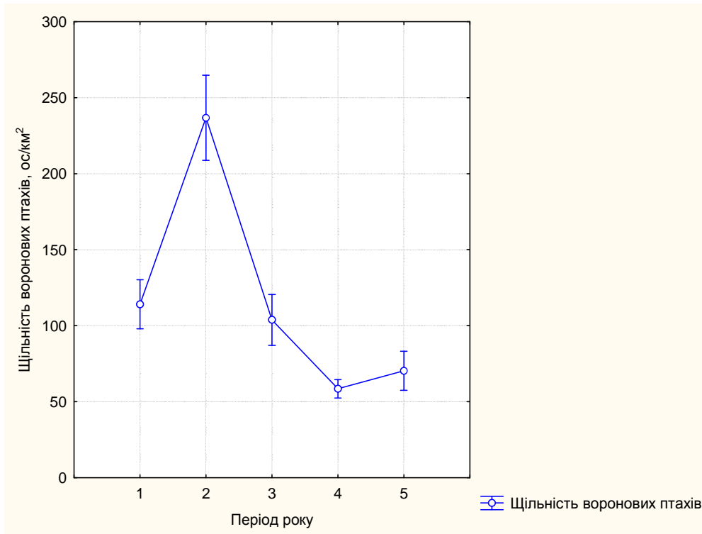
Рис. 1. Динаміка щільності воронів у м. Житомирі за періодами року
