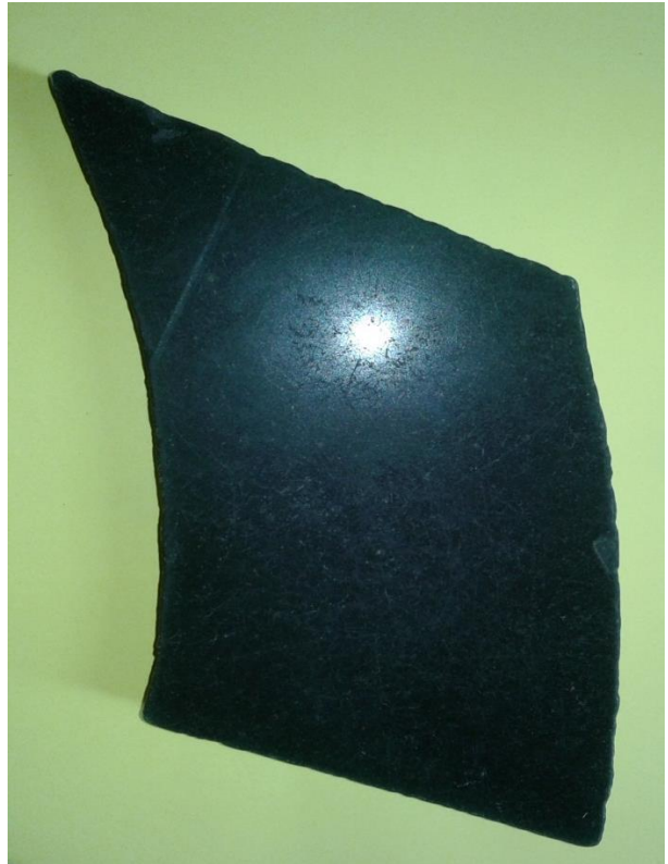
Рис. 1.10. Плита базальту
