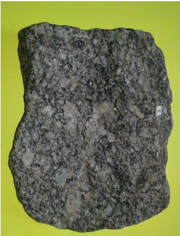
Рис. 1.19. Граніт
