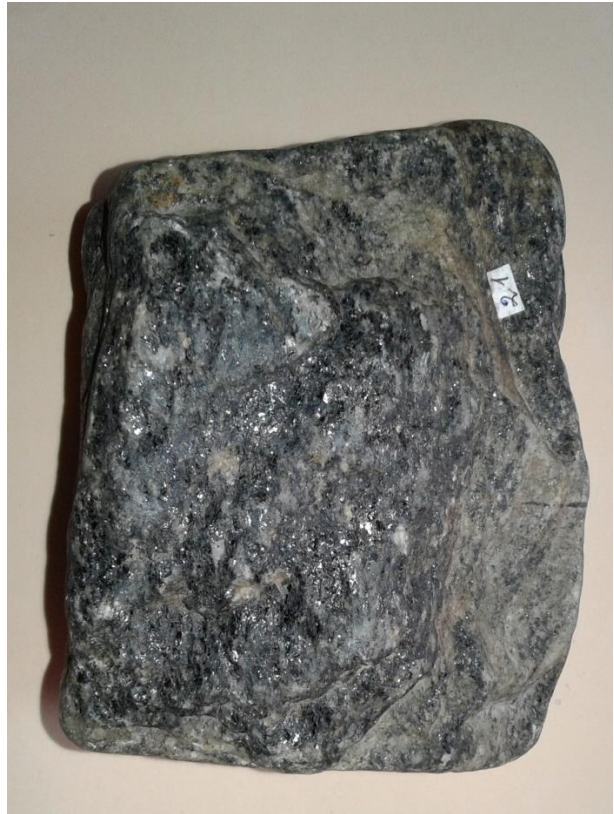
Рис. 3.14. Хлоритовий сланець
