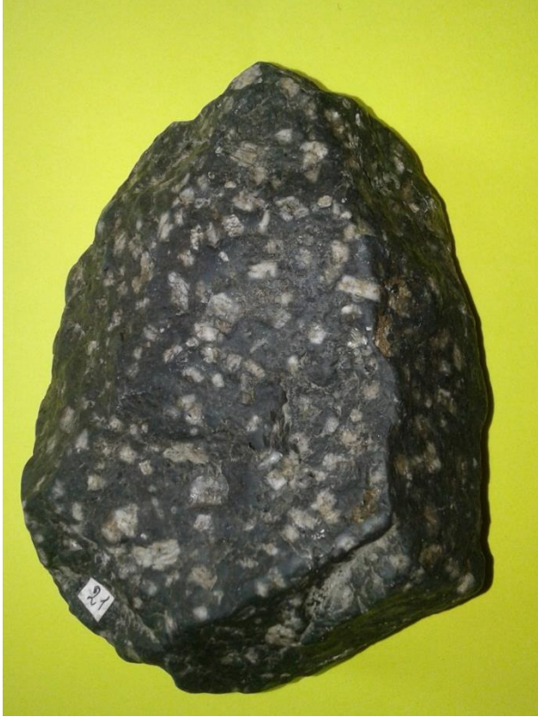
Рис. 1.13. Діорит
