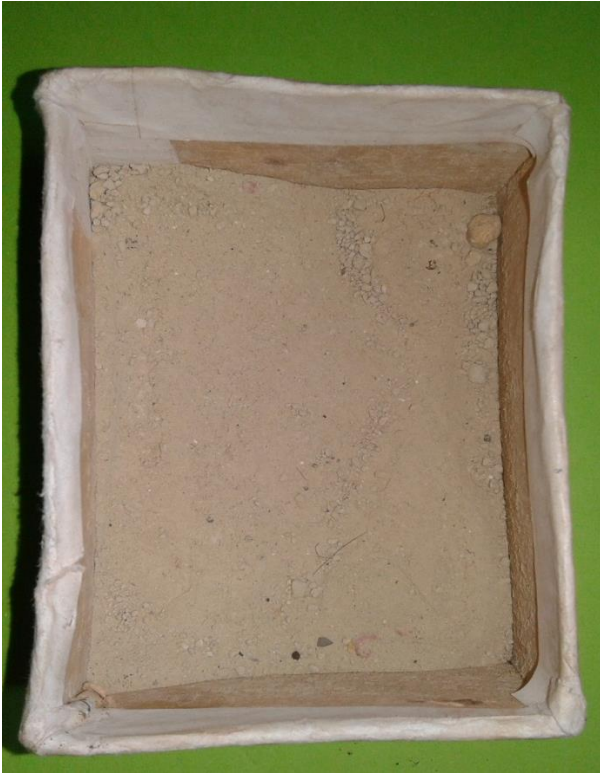
Рис. 2.13. Лес
