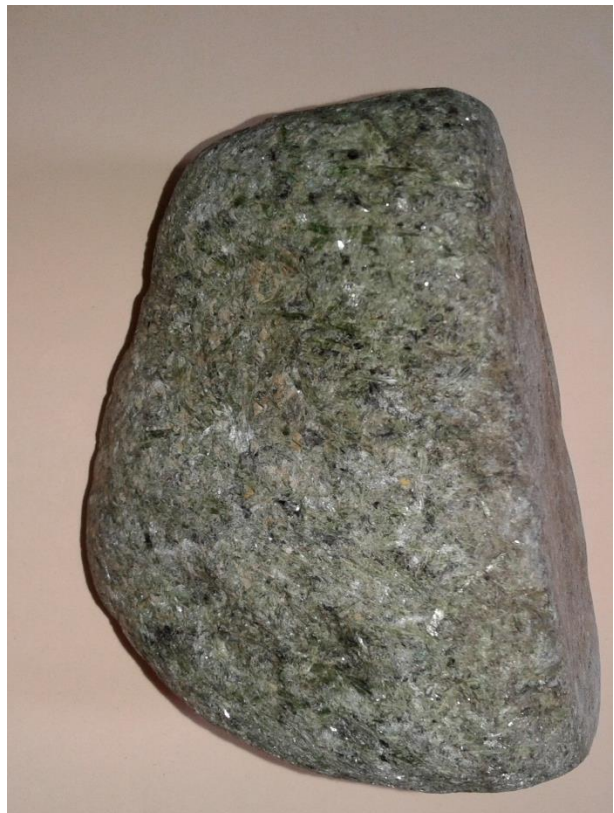
Рис. 3.16. Актинолітовий сланець
