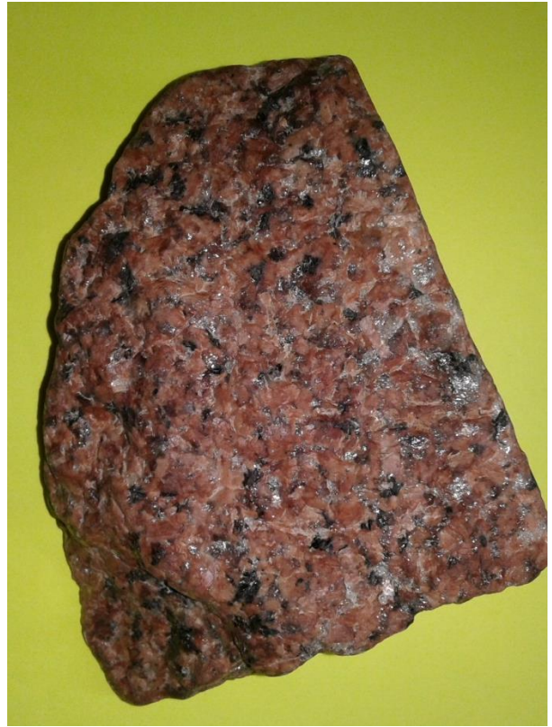
Рис. 1.18. Граніт
