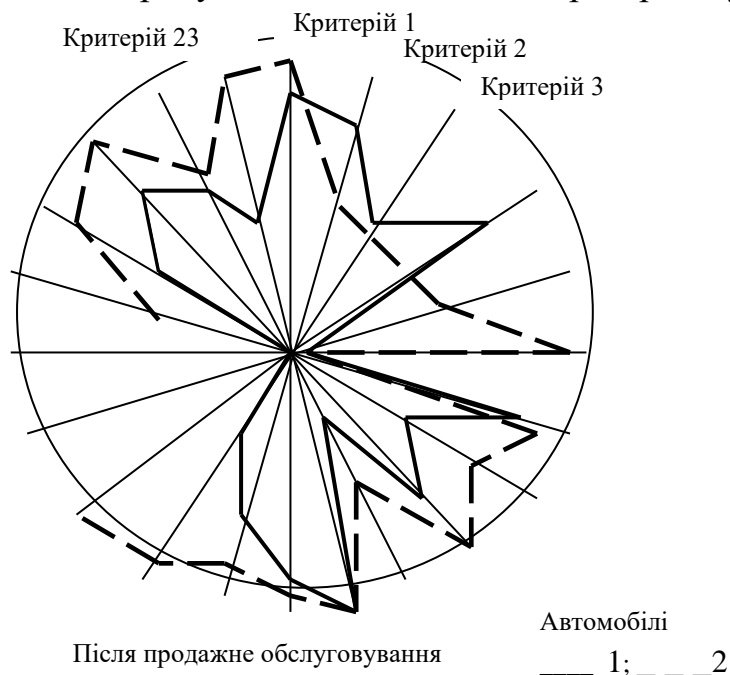
Рис. 5.1. Радар конкурентоспроможності
