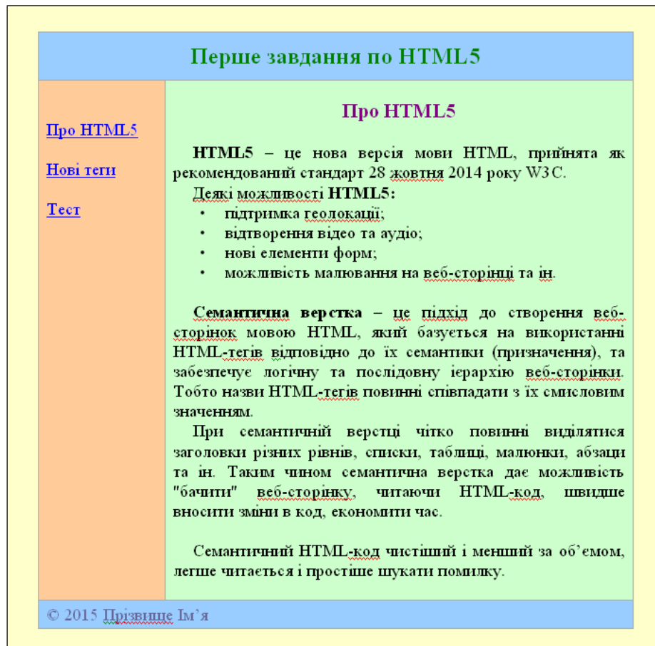
Рисунок 16 – Приклад верстки
