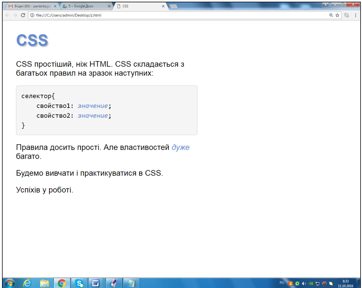
Рисунок 15 – Зразок веб-сторінки
